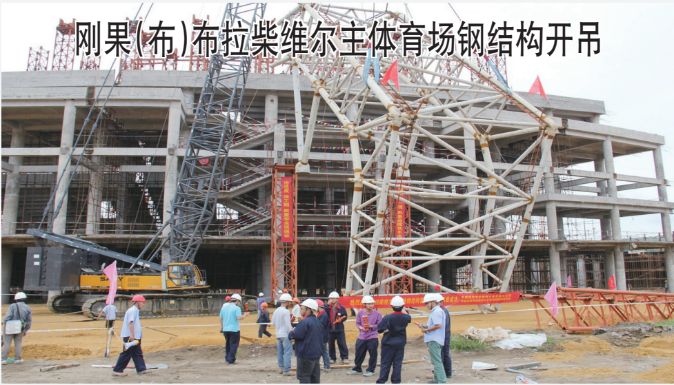
刚果(布)布拉柴维尔主体育场钢结构开吊 近日,随着重达83吨的双拱墙面段钢桁架被徐徐吊起并安装就位,中国建筑承建的刚果(布)布拉柴维尔体育场项目主体育场钢结构吊装施工正式开始。该项目是2015年第十一届全非洲运动会场地。 (胡兴良/摄影报道)
