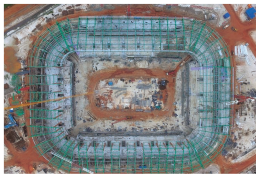
近日,由中建安装具体实施的加蓬让蒂尔港体育场钢结构主桁架吊装工程提前完成,其环向桁架结构罩棚,长201米宽161米,施工工况复杂。让蒂尔港体育场是2017年第31届非洲杯足球赛分赛场。(彭影 刘杰杰)
