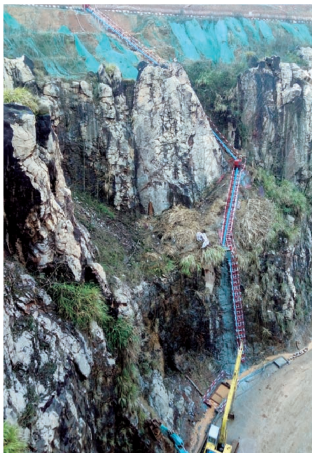
近日,中建五局承建、中建西部建设湖南公司供应混凝土的长沙湘江欢乐城项目,深坑混凝土大落差溜管输送新工艺获得圆满成功,其高达百米的落差,刷新了国内混凝土原向下输送77米的深度记录。(刘小峰 胡小波)
