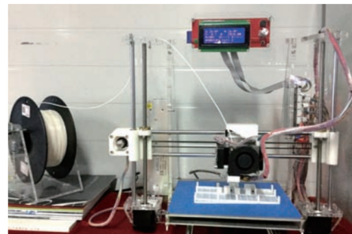
存在关键施工点楼层的实体模型在3D打印机的有序运作下,慢慢成形。
