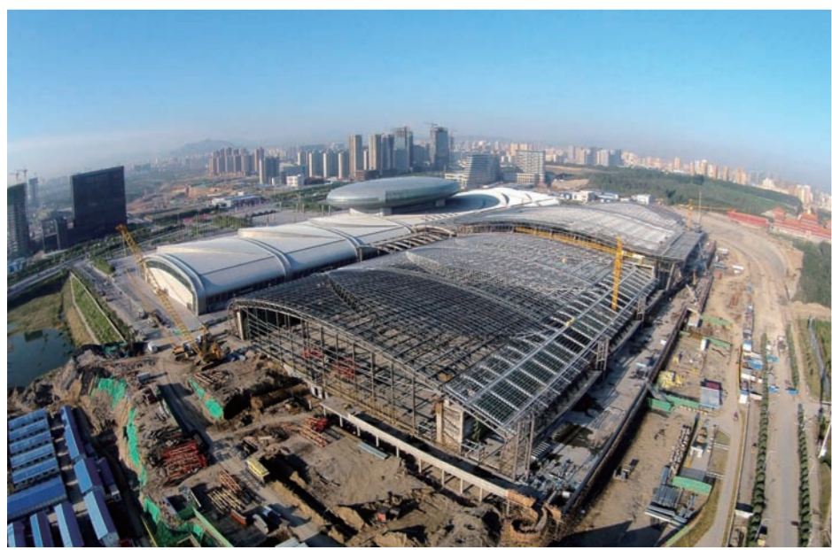
近日,由中建三局西北公司承建、位于乌鲁木齐市、总建筑面积约20万平方米的新疆国际会展中心二期项目钢结构主体封顶。(李涛 赵雯婷)
